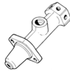
1201 Hoofdrempomp 17 mm enkel circuit Hauptbremszylinder 17 mm, Einkreis • Typ(e) 1/Typ(e)14 08/65-07/67
