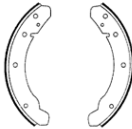
1230 Remschoenen 230 x 40 Vooraan Type 1 08/64- Achteraan Type 1 1200 11/67- 13/15/1600 08/67- 1302/03 Bremsbacken 230 x 40 Vorne Typ 1 08/64- Hinten Typ 1 1200 11/67- 13/15/1600 08/67- 1302/03
