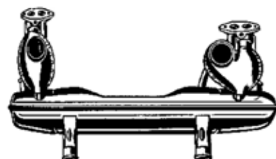
1052 Uitlaat met dubbele voorverwarming Auspuff mit doppelter Vorwärmung • Typ(e) 1 code AR/AS
