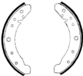
1232 Remschoenen 230 x 40 Vooraan Type 1/ Type 14 08/57-07/64 Bremsbacken 230 x 40 Vorne Typ 1/ Typ 14 08/57-07/64
