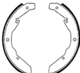
1237-1 Remschoenen 250 x 46 Achteraan Type 2 08/63-07/70 Bremsbacken 250 x 46 Hinten Typ 2 08/63-07/70
