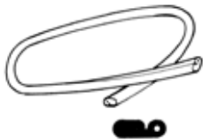
0751 Rubber dichting tussen luchtinlaatrooster en binnenspatbord, vooraan, per paar Dichtung zwischen Lufteinlassgitter und Frontmaske, Paar • 08/59-07/74
